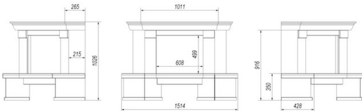
Obudowa wkładu kominkowego narożna Maja/Antek
